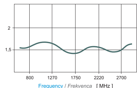
VSWR
